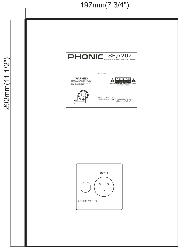
SE207 / SEp207 Back Panel SE207 / SEp207 Panel Trasero SE207 / SEp207 后面板
